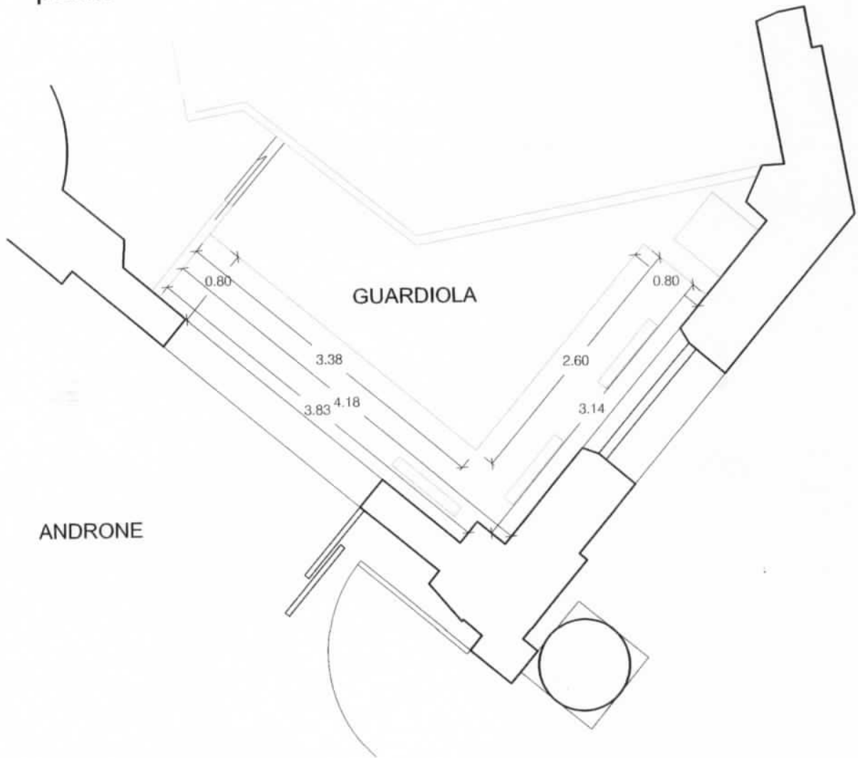
DETTAGLIO GUARDIOLA (81) scala 1:50 pianta
